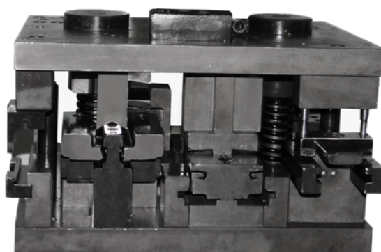
PUNZÓN 8 ESTACIONES COLOSAL 2.6 PUN COL8
