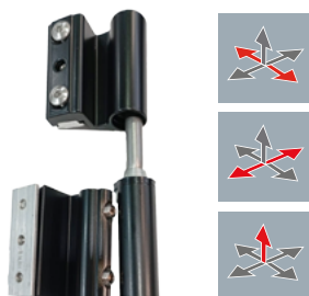
BISAGRA 2 ALETAS REGULABLE NEGRA PARA 120 KILOS SIDERAL/TAIRONA
