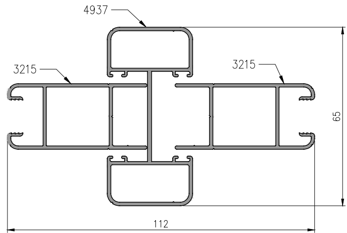
EXTERIOR Sección A-A' Escala 1:1
